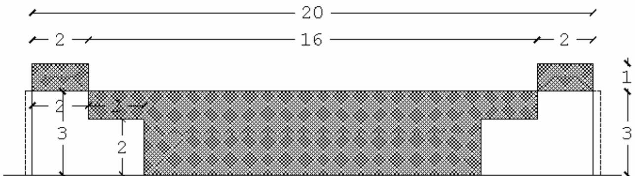
VARIANTE 1 (dimensiones interiores)
